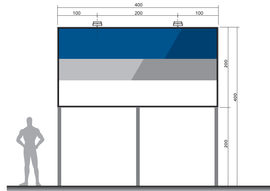
ILUMINAÇÃO FRONT LIGHT REFLETOR LÂMPADA HALÓGENA 500W
